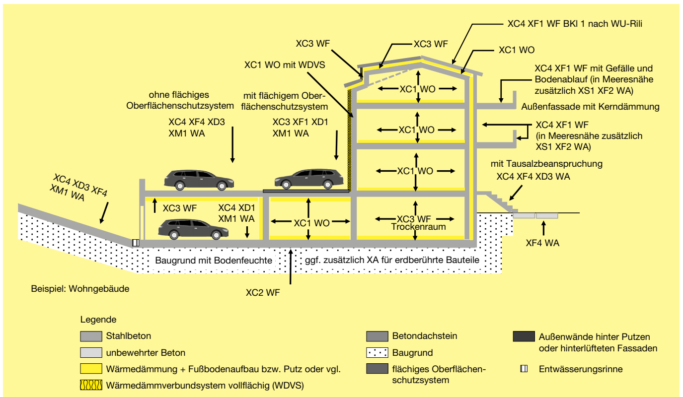
Bild 1: Beispiel für mehrere, gleichzeitig zutreffende Expositionsklassen an einem Wohnhaus
