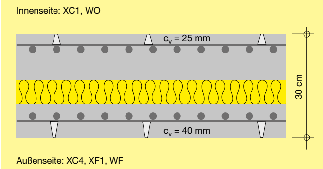
Bild 3: Ortbetonwand mit Kerndämmung C25/30, Längs- und Querbewehrung \Phi 14 mm (ohne Anforderungen an den Brandschutz)
